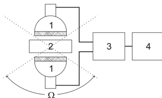
Рис.3 Блок-схема установки.
